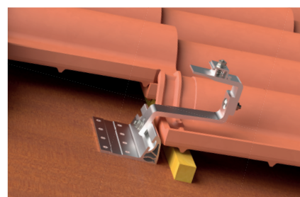
Dettaglio: gancio in alluminio GTA3.
